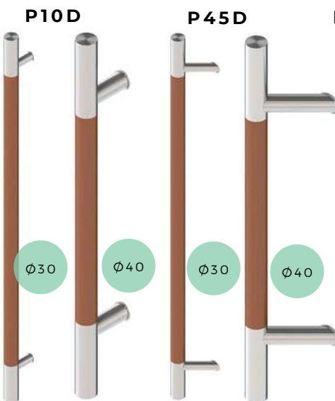
P10D und P45D Türgriffe: Länge: 600-1600mm
