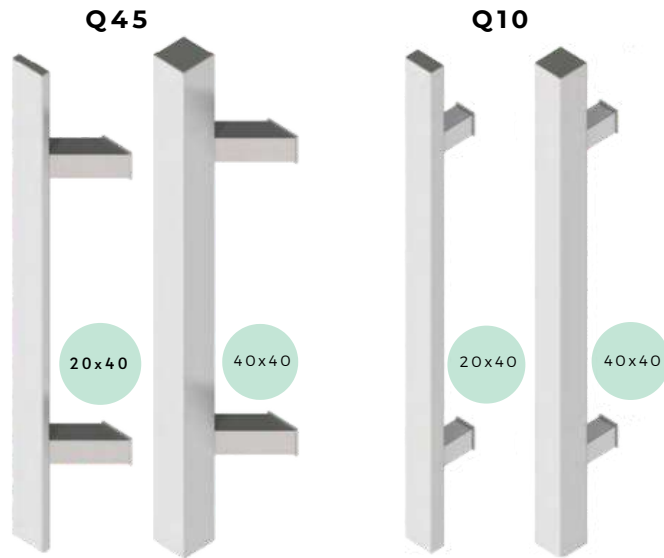
Türgriffe Q45 und Q10: Standardlänge 300-1800mm Individuelle Länge: 1801-2200mm - gegen Aufpreis: 110 EUR (über 1800mm nur Option 40x40 möglich) Farben: Edelstahl oder RAL-Palette
