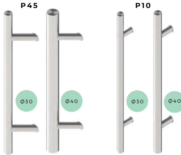
Türgriffe P45 und P10: Standardlänge 300-1800mm Individuelle Länge: 1801-2200mm - gegen Aufpreis 110 EUR (über 1800mm nur Option Ø40 möglich) Farben: Edelstahl oder RAL-Palette
