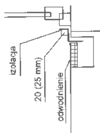
Rys. 36. Dopuszczalna wysokość progu w mieszkaniach dla niepełnosprawnych, poruszających się na wózkach inwalidzkich
