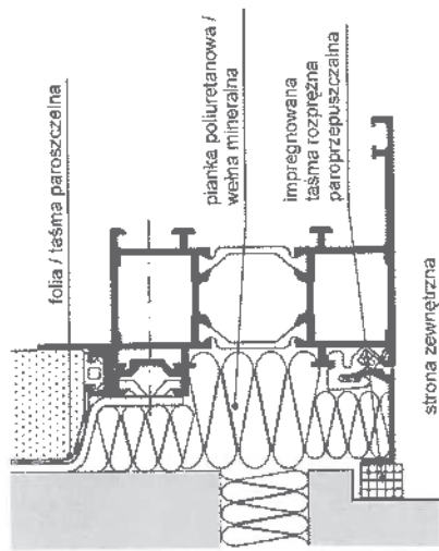
Rys. Z2-2. Przykład uszczelnienia szczytliny między oknem aluminiowym a ościeżem bez węgarka w ścianie trójwarstwowej z izolacją w środku
