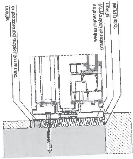
Rys. Z2-14. Przykład uszczelnienia aluminiowych drzwi balkonowych przesuwnych w ścianie dwuwarstwowej z ocieplaniem zewnętrznym. Przekrój poziomy
