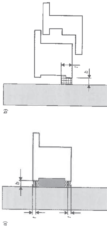
Rys. 30. Wymiary uszczelnienia: a) z kitu trwale elastycznego, b) z impregnowanych rozprężnych taśm paroszczelnych
